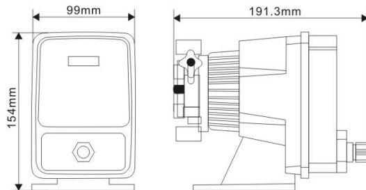
Dimensional 尺寸图
